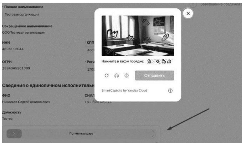
Рисунок 3 - Проверка CAPTCHA
